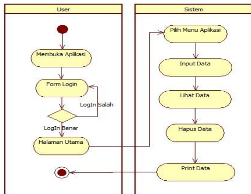
Gambar 5 : Activity Diagram Login Aplikasi
